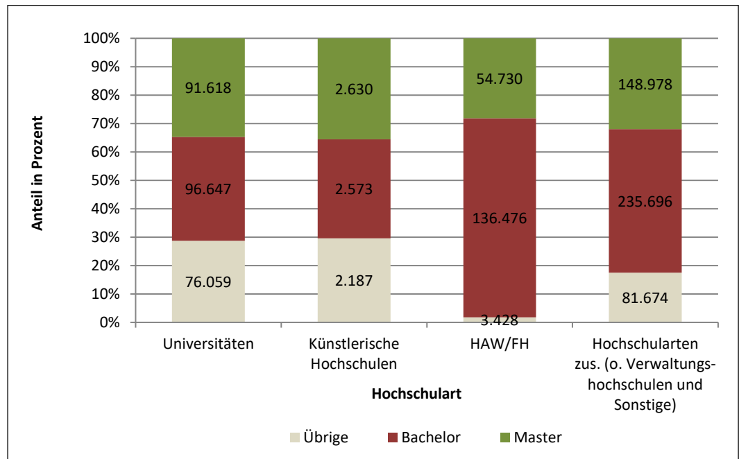
Diagramm 3.2 Bestandene Prüfungen nach Hochschularten und Prüfungsgruppe im Prüfungsjahr 2024
