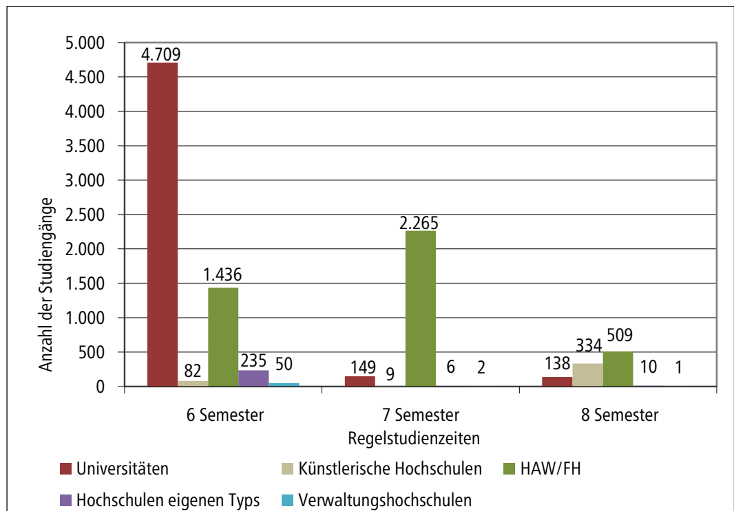
Diagramm 1.6.1 Regelstudienzeiten in den Bachelorstudiengängen nach Hochschularten im Wintersemester 2025/2026
