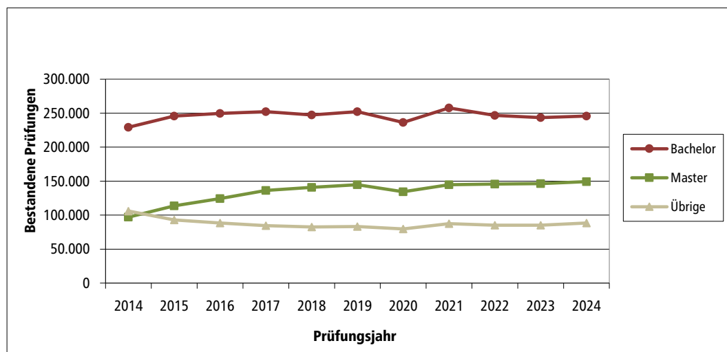
Diagramm 3.1 Bestandene Prüfungen nach Prüfungsgruppen Bachelor, Master und Übrige, Prüfungsjahr 2014 bis Prüfungsjahr 2024
