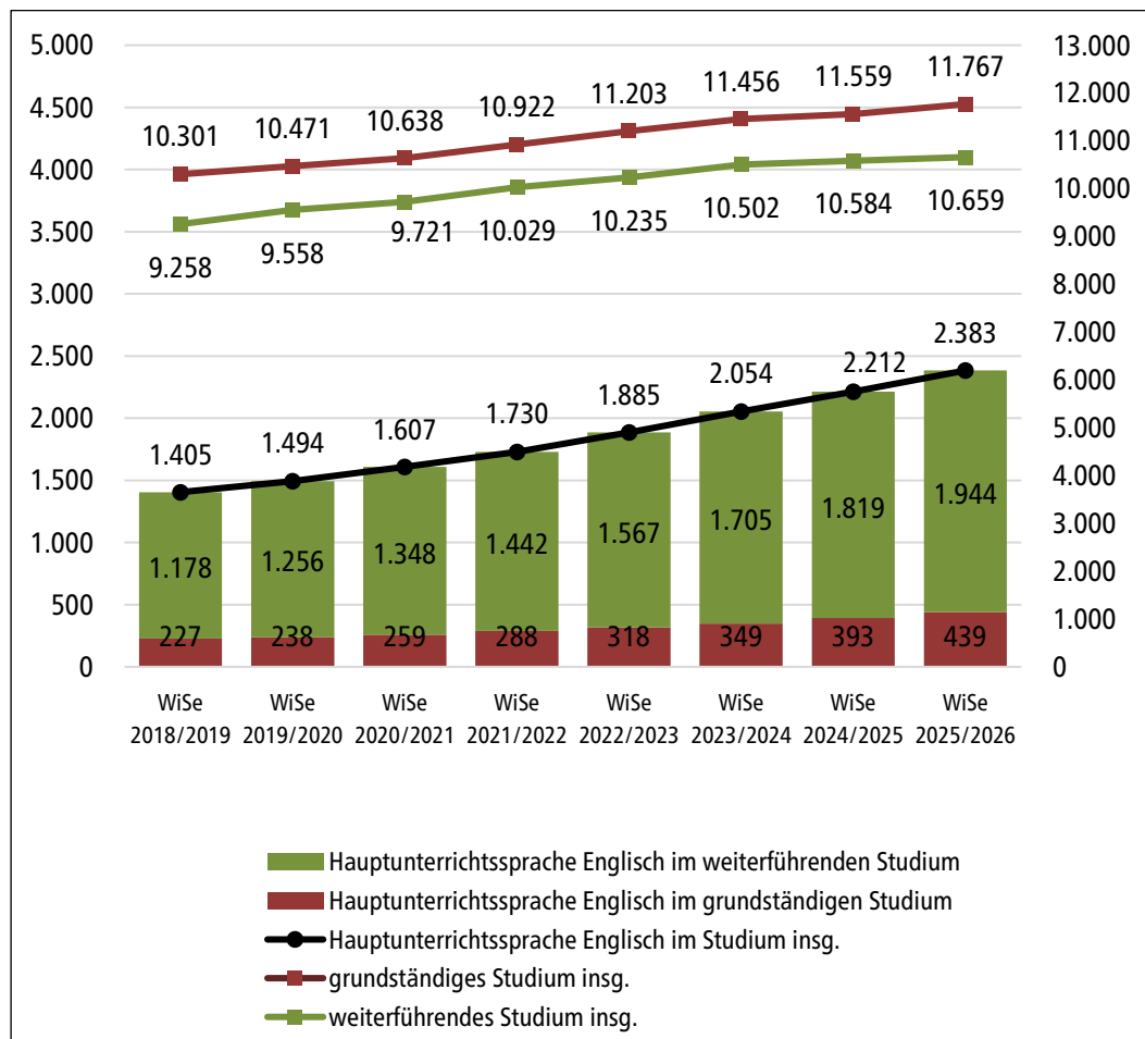
Diagramm 1.10 Entwicklung der Studiengänge mit Hauptunterrichtssprache Englisch
