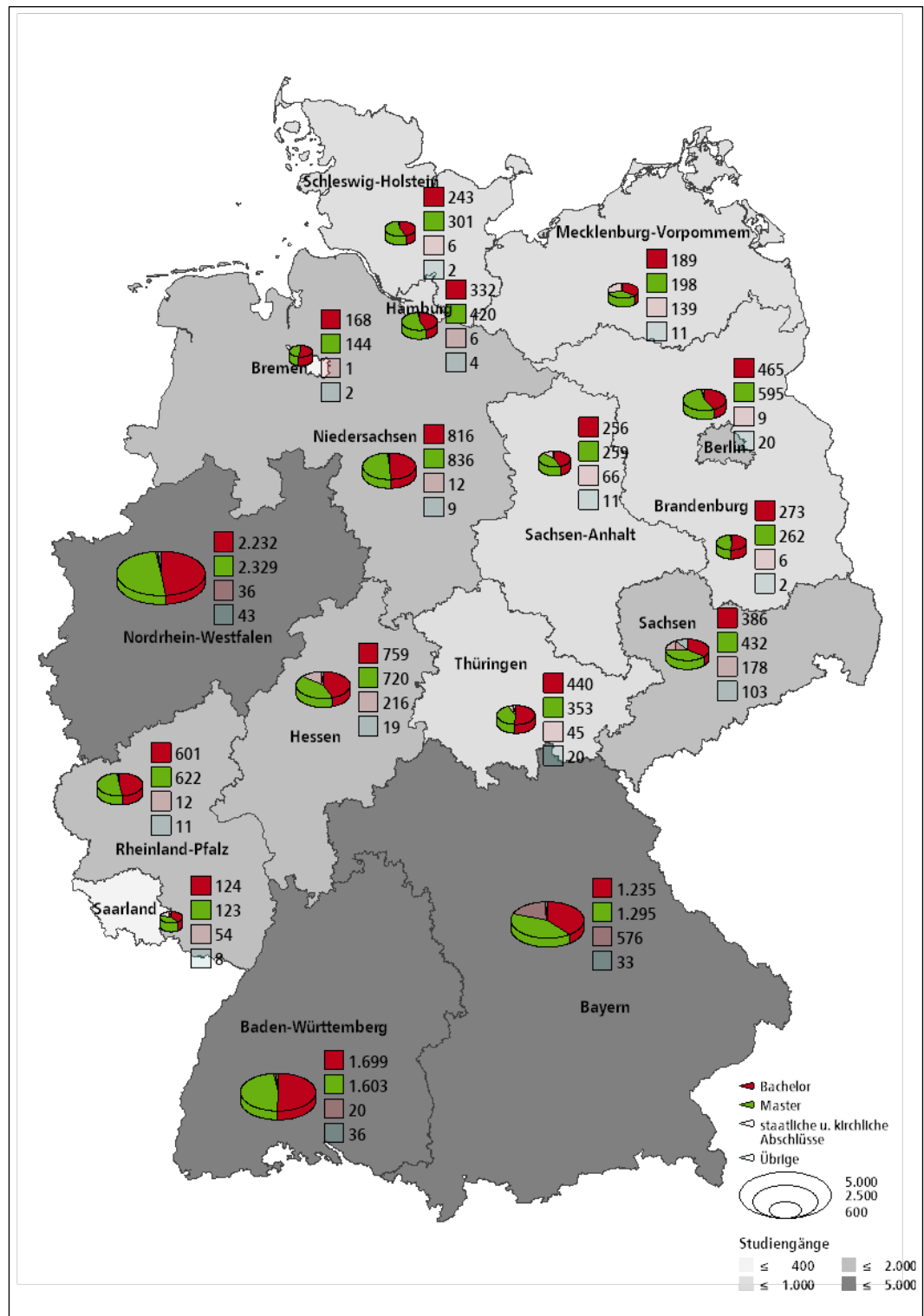
Karte 1.5 Studienangebote nach Bundesländern im Wintersemester 2025/2026
