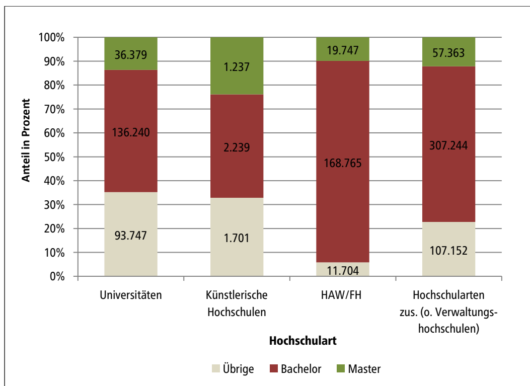
Diagramm 2.2.1 Studienanfänger:innen im 1. Hochschulsesemester nach Hochschulart und angestrebten Prüfungsgruppen Bachelor, Master und Übrige im Studienjahr 2024
