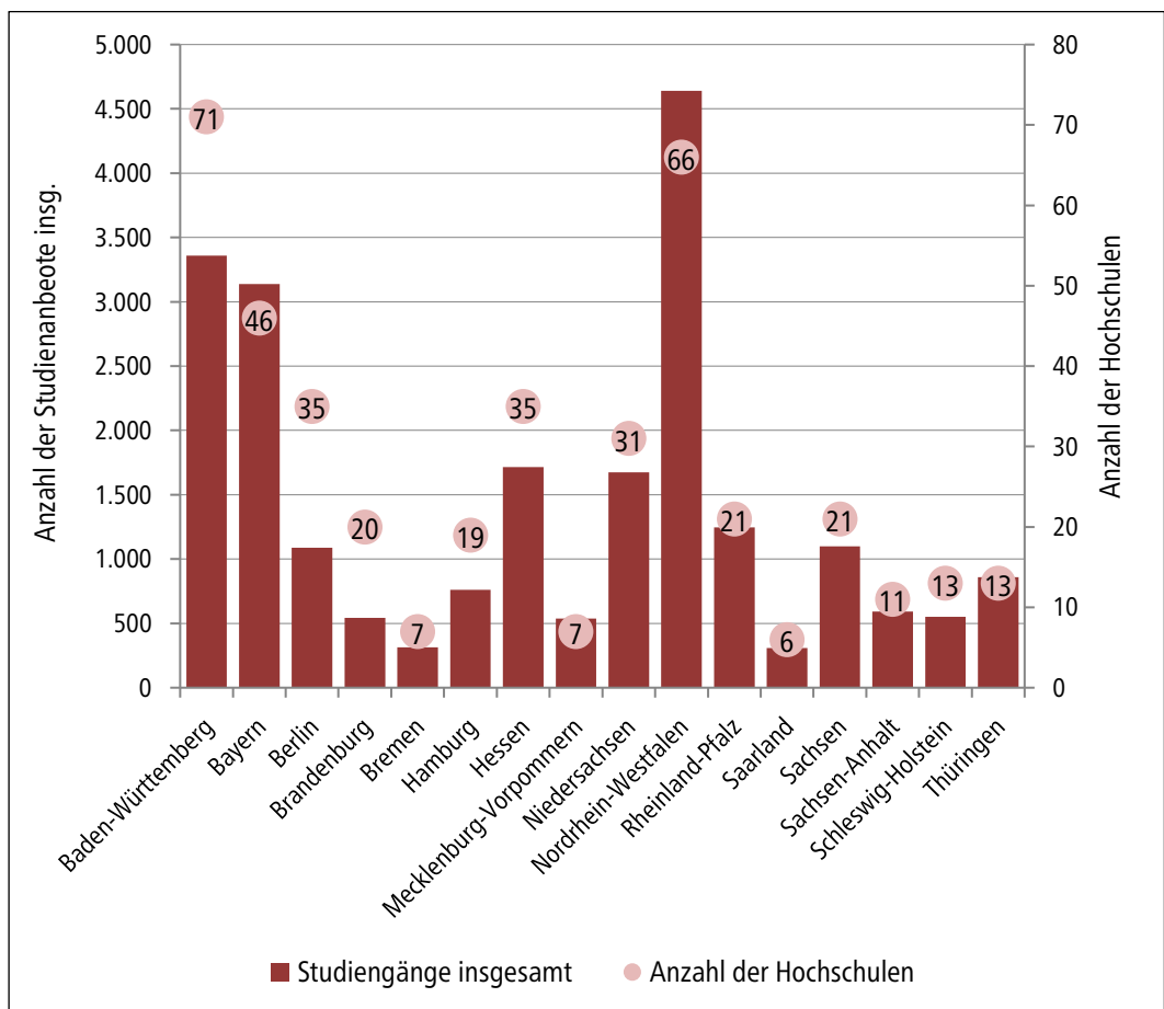
Diagramm 1.5 Studienangebote nach Bundesländern im Wintersemester 2025/2026
