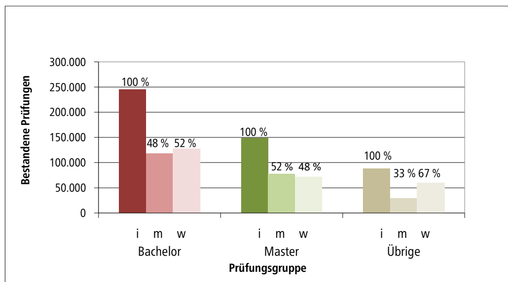
Diagramm 3.3 Bestandene Prüfungen nach Geschlecht in den Prüfungsgruppen Bachelor, Master und Übrige im Prüfungsjahr 2024
