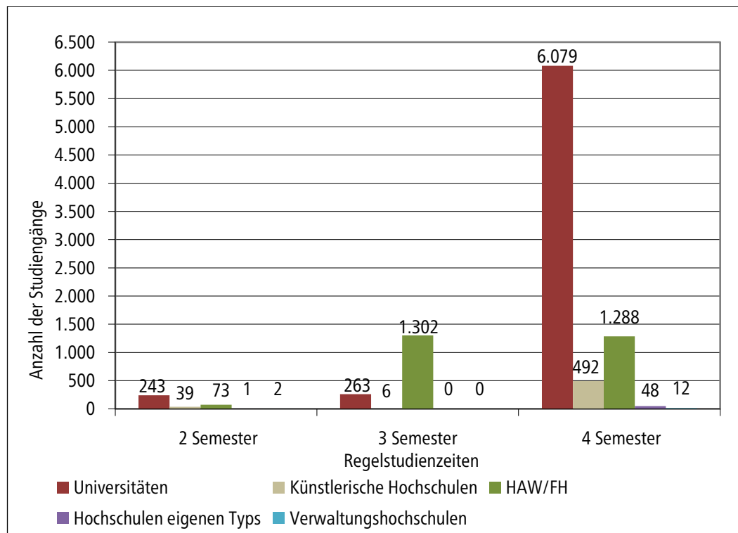
Diagramm 1.6.2 Regelstudienzeiten in den Masterstudiengängen nach Hochschularten im Wintersemester 2025/2026
