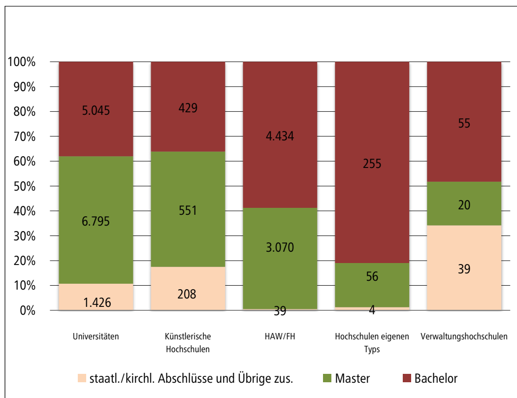
Diagramm 1.2 Studienangebote nach Hochschularten und Abschlussarten im Wintersemester 2025/2026
