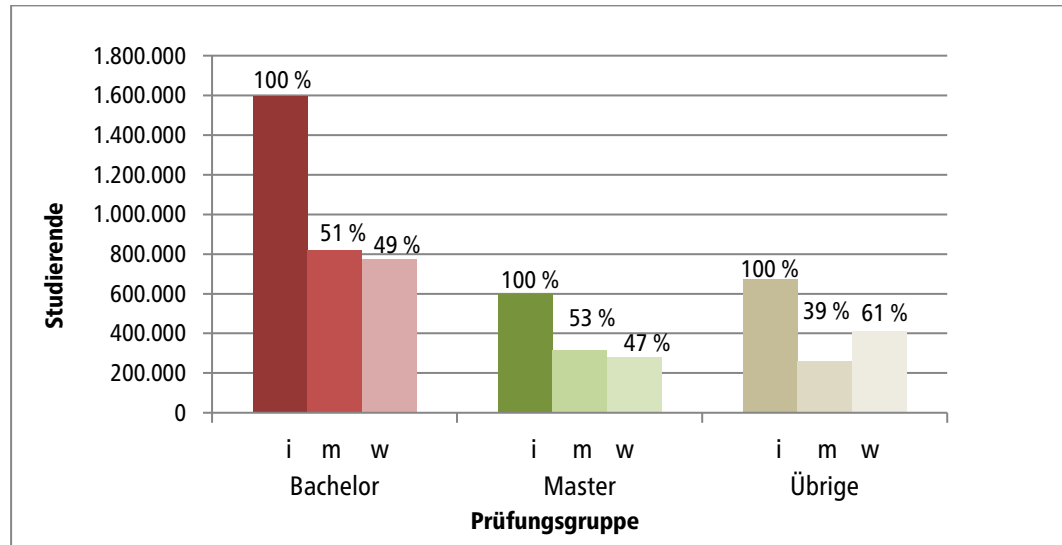
Diagramm 2.3 Studierende nach angestrebten Prüfungsgruppen Bachelor, Master und Übrige nach Geschlecht im Wintersemester 2024/2025
