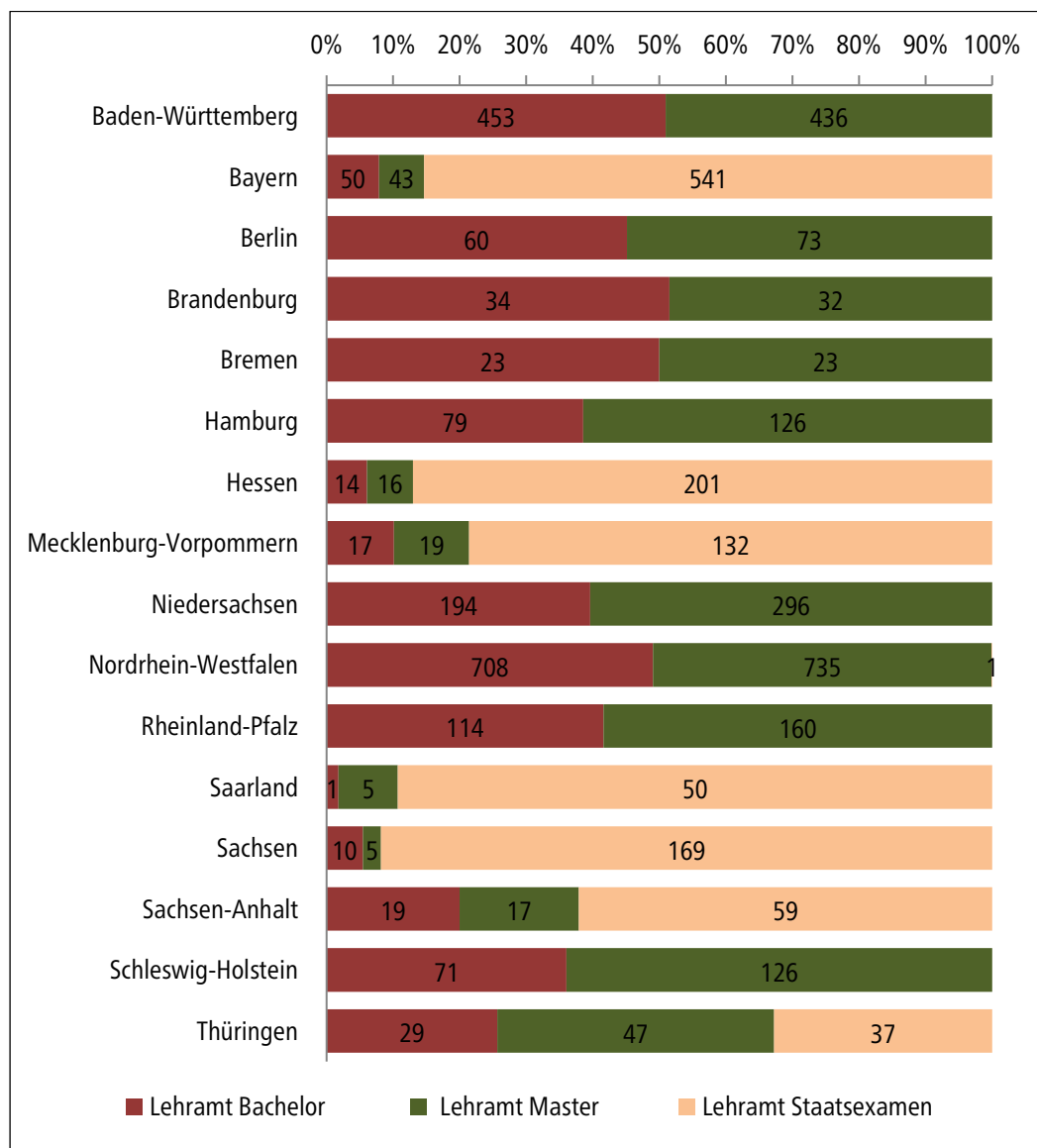
Diagramm 1.4 Studienangebote in der Lehrer:innenbildung im Wintersemester 2025/2026
