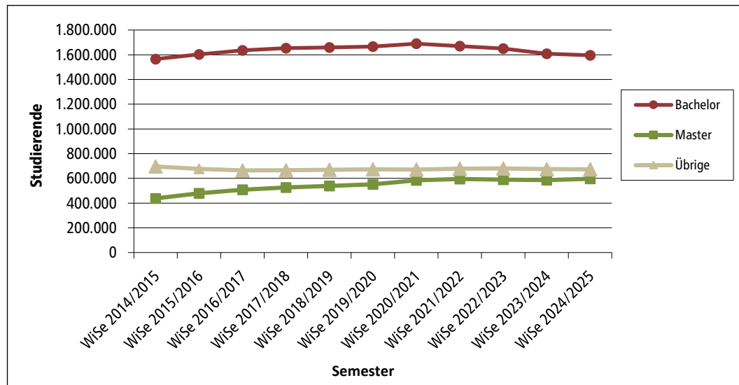
Diagramm 2.1.1 Studierende nach angestrebten Prüfungsgruppen Bachelor, Master und Übrige, Wintersemester 2014/2015 bis Wintersemester 2024/2025
