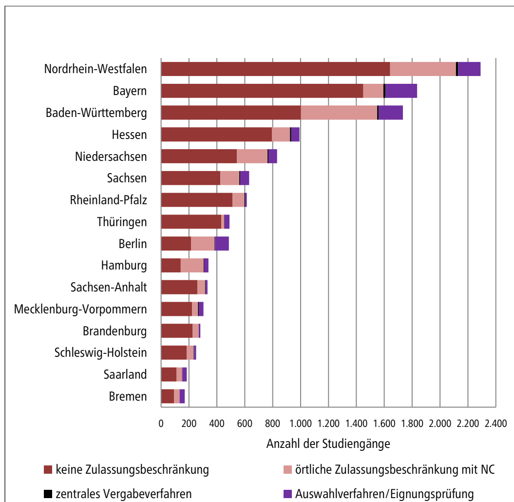
Diagramm 1.8 Zulassungsmodi der grundständigen Studiengänge nach Bundesländern im Wintersemester 2025/2026
