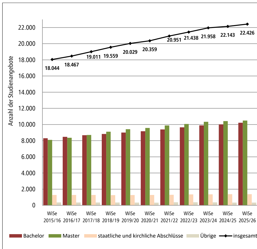
Diagramm 1.1 Entwicklung der Studienangebote, Wintersemester 2015/2016 bis Wintersemester 2025/2026
