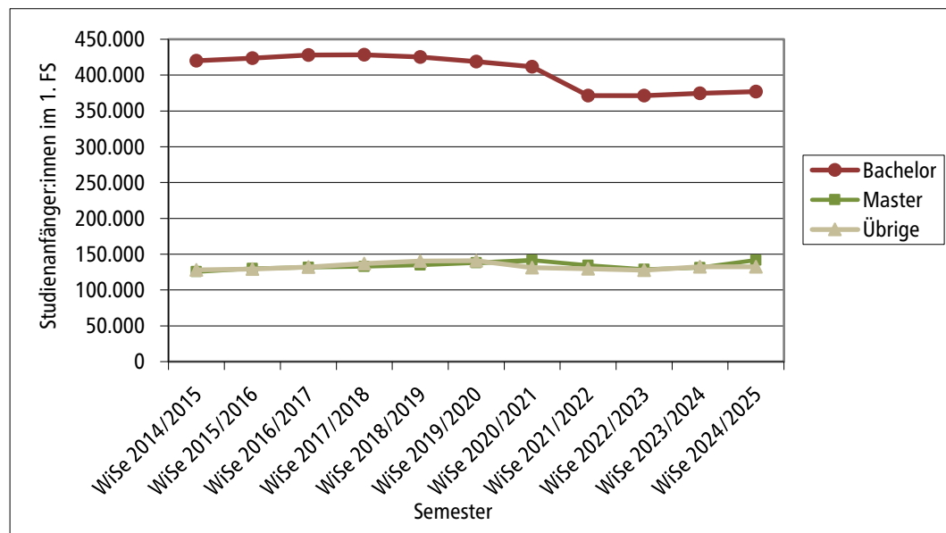
Diagramm 2.1.3 Studienanfänger:innen im 1. Fachsemester nach angestrebten Prüfungsgruppen Bachelor, Master und Übrige, Wintersemester 2014/2015 bis Wintersemester 2024/2025
