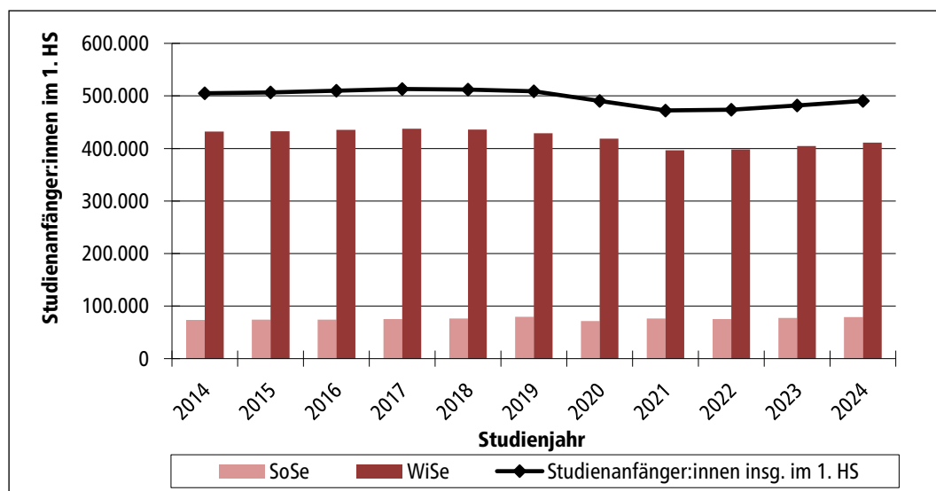
Diagramm 2.1.2 Studienanfänger:innen im 1. Hochschulsemester in den Studienjahren 2014 bis 2024 insgesamt, Sommersemester und Wintersemester
