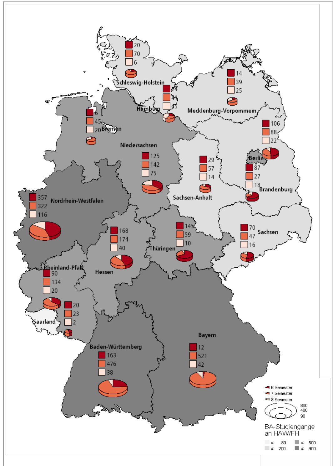
Karte 1.6 Bachelorstudiengänge an HAW/FH nach Regelstudienzeit im Wintersemester 2025/2026
