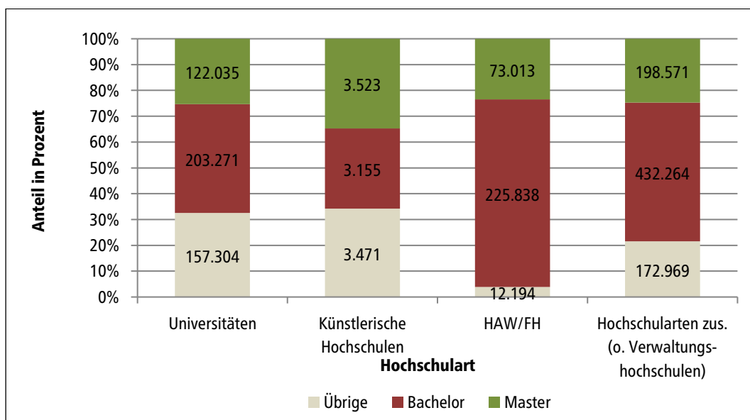
Diagramm 2.2.2 Studienanfänger:innen im 1. Fachsemester nach Hochschularten und angestrebten Prüfungsgruppen Bachelor, Master und Übrige im Studienjahr 2024
